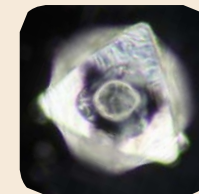
Dunkelfeld
