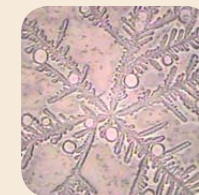
Kristallanalyse
